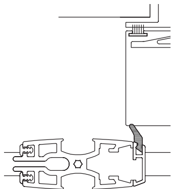
Sello de espuma Q-Lon (QL7066)
