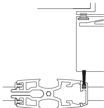
Sello de cepillo (SEL-042)
