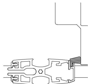
Sello de espuma Q-Lon (AQ109)
